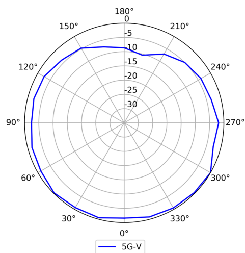
5GHz (垂直)
