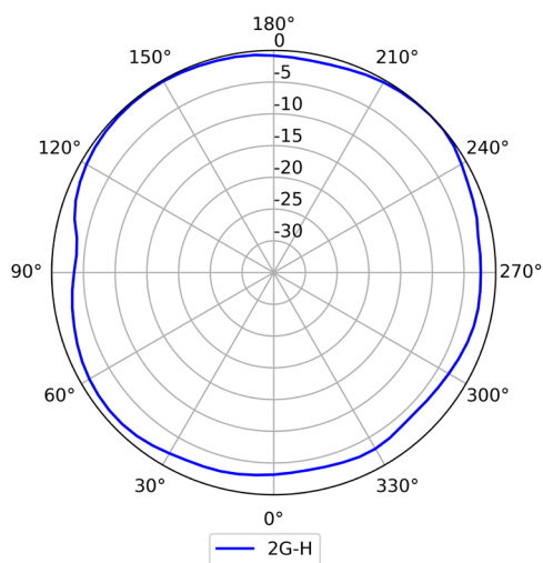
2.4GHz (水平)
