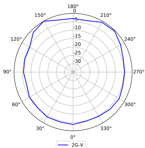
2.4GHz (垂直)
