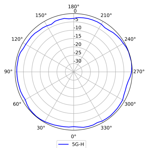
5GHz (水平)
